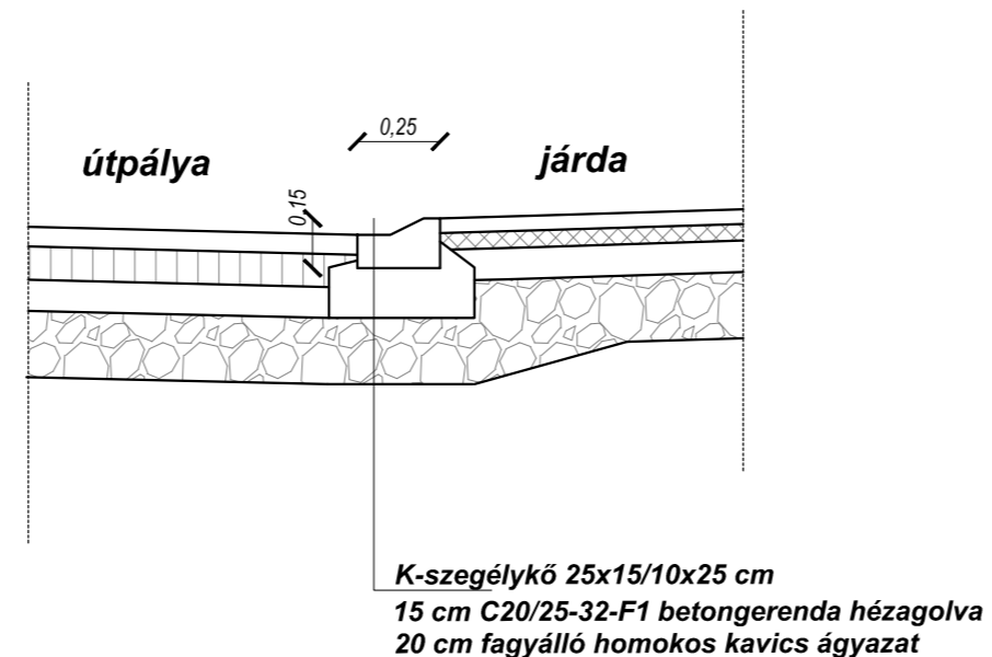
RÉSZLETRAJZ K SZEGÉLYKŐ METSZET M=1:25
