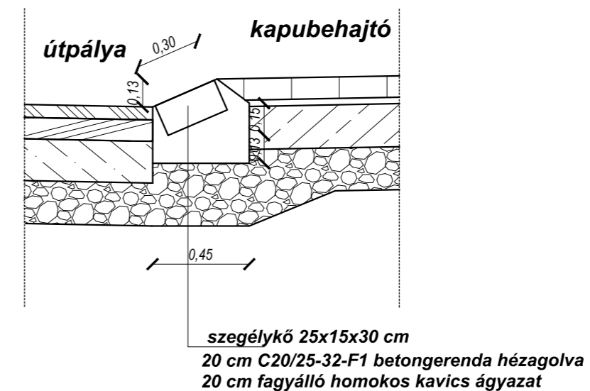
RÉSZLETRAJZ DÖNTÖTT SZEGÉLYKŐ METSZET M=1:25
