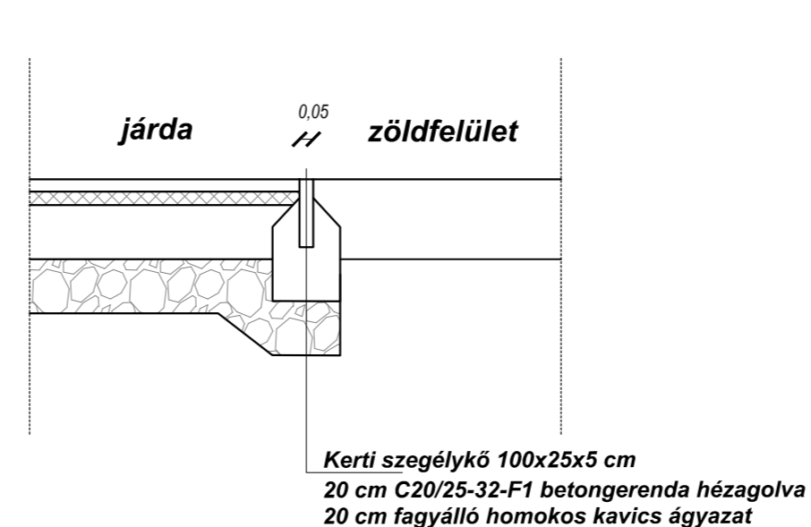
RÉSZLETRAJZ KERTI SZEGÉLYKŐ METSZET M=1:25
