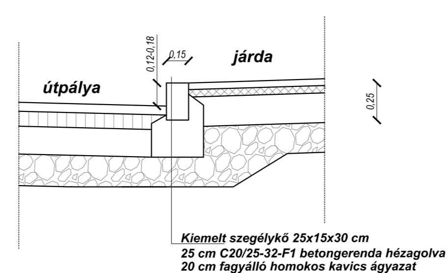
RÉSZLETRAJZ KIEMELT SZEGÉLYKŐ METSZET M=1:25
