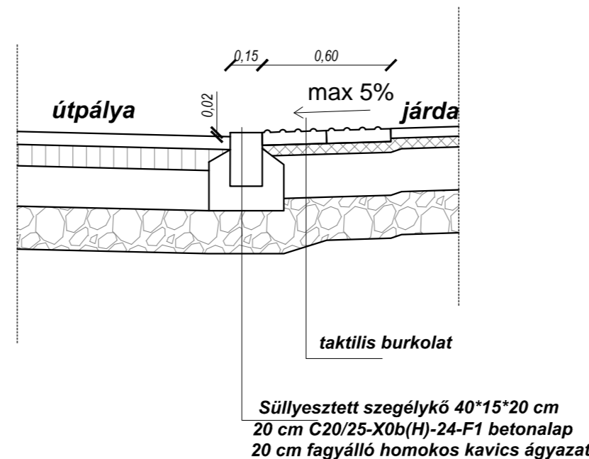
RÉSZLETRAJZ SZEGÉLYSÜLLYESZTÉS METSZET M=1:25
