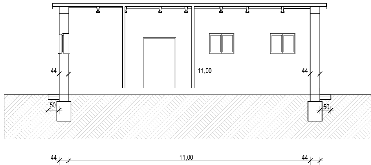
5B-5B Metszet
