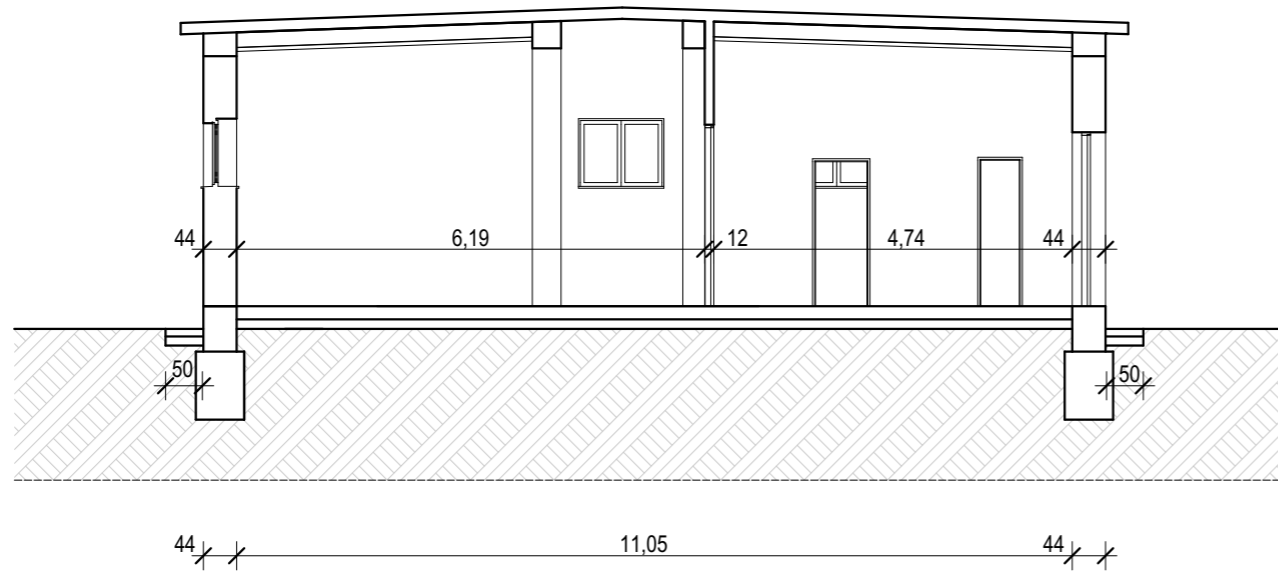
5A-5A Metszet
