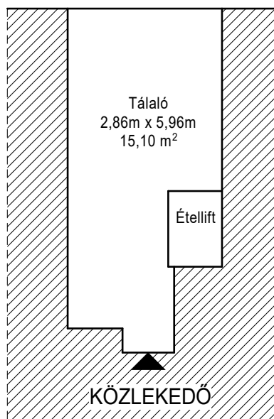
EMELETI ALAPRAJZ
