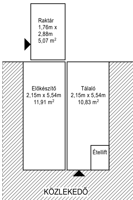
FÖLDSZINTI ALAPRAJZ
