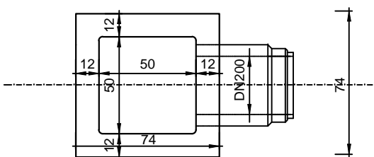
A-A metszet
