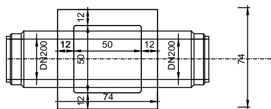
A-A metszet
