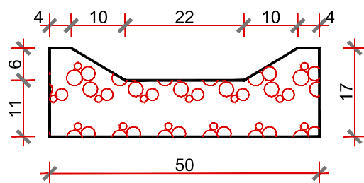
KERESZTMETSZET
