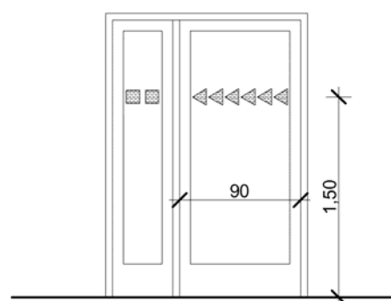
AJTÓK JELÖLÉSE M=1:50
